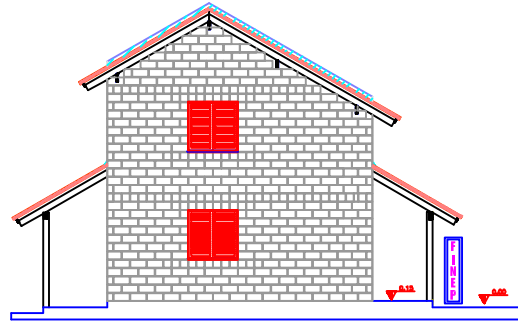
Fachada Lateral Protótipo de Blocos de Concreto ESC: 1/50
