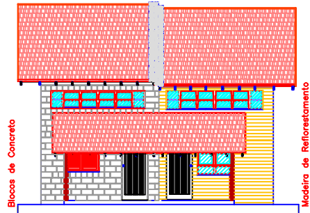
Fachada Frontal Protótipos Geminados ESC: 1/50
