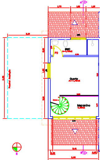
Planta Baixa do Pavto. Superior
