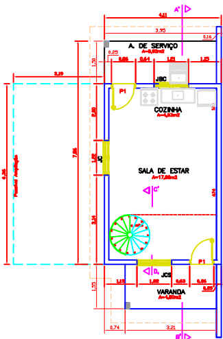
Planta Baixa do Térreo
