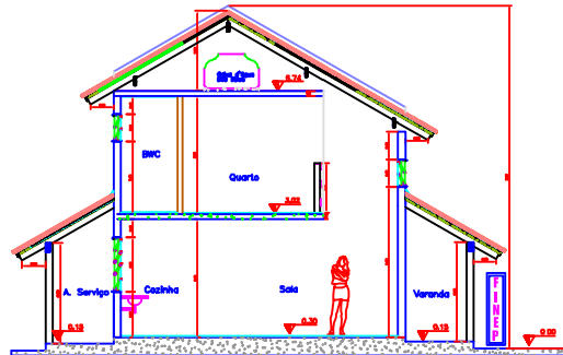
Corte do Protótipo de Blocos- A'B' ESC: 1/50
