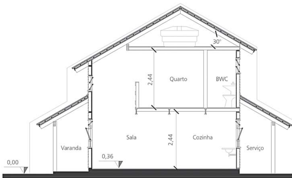
Figura 3: Corte longitudinal
