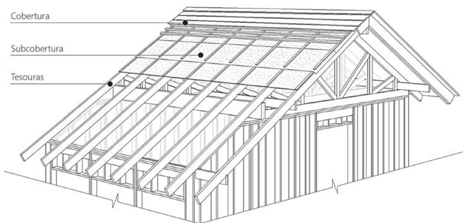
Figura 28: Subsistema telhado
