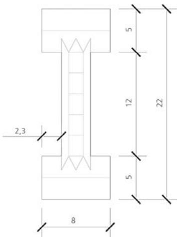
Figura 20: Viga “I”
