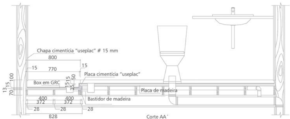
Figura 36: Corte longitudinal da laje do banheiro
