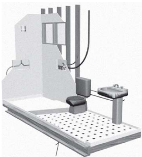
Figura 47: Vista do banheiro com seus componentes industrializados
