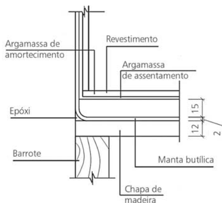
Figura 49: Box com chapa de madeira e manta butílica
