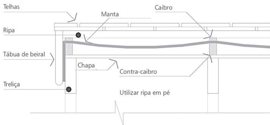
Figura 33: Camada de ar entre chapa e manta
