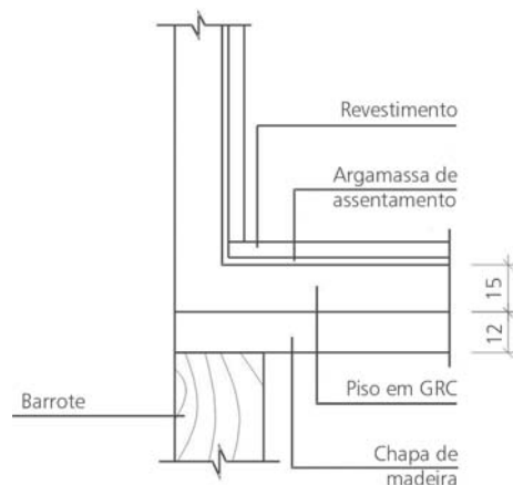
Figura 48: Box em GRC e revestimento cerâmico
