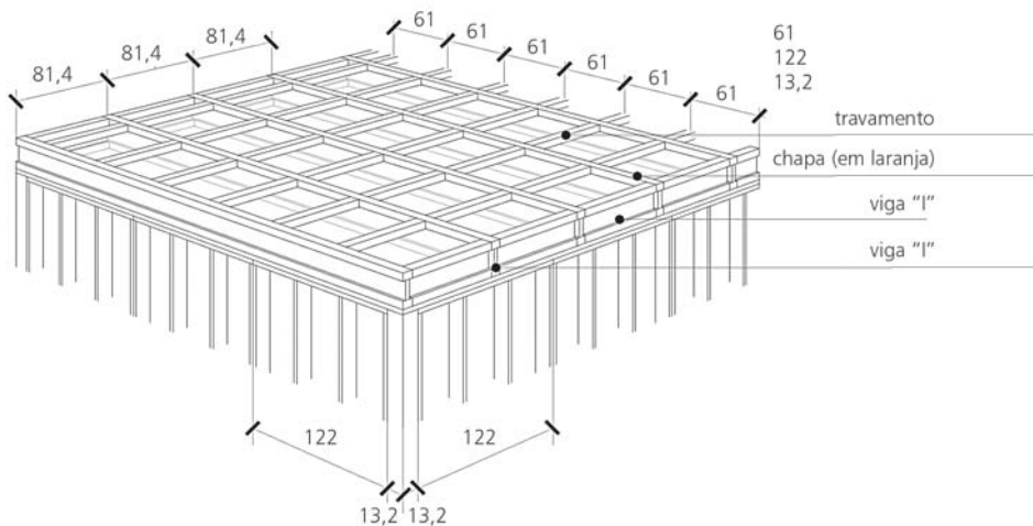
Figura 25: Modulação proposta para o entrepiso
