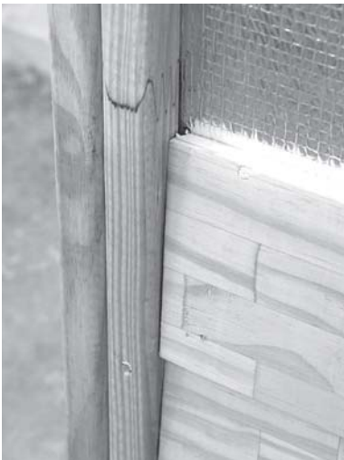
Figura 17: Encontro entre o siding e o acabamento de canto
