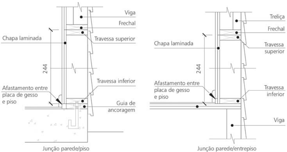
Figura 13: Detalhe proposto para a junção entre parede, piso e entrepiso
