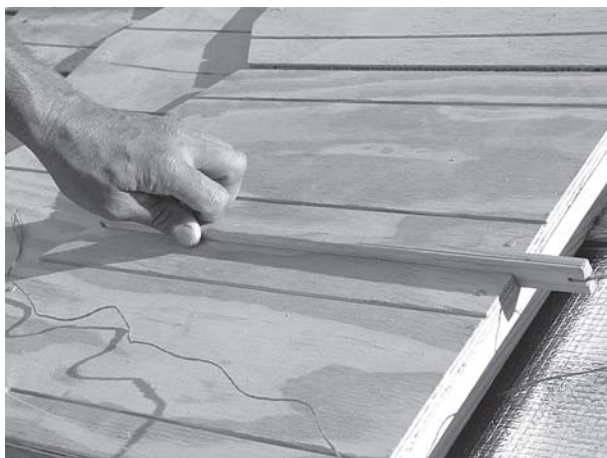
Figura 30: Utilização de gabarito para espaçamento das telhas
