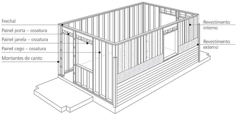
Figura 10: O subsistema parede
