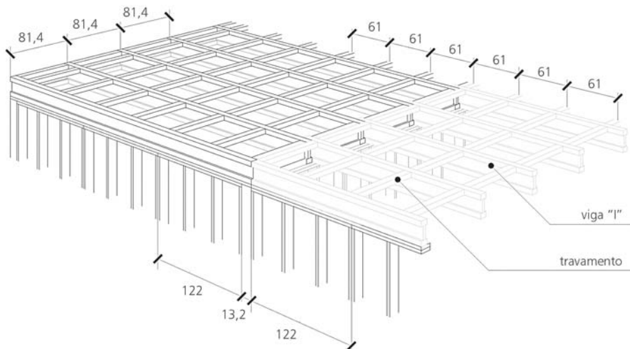
Figura 27: Estrutura do entrepiso no caso de ampliação
