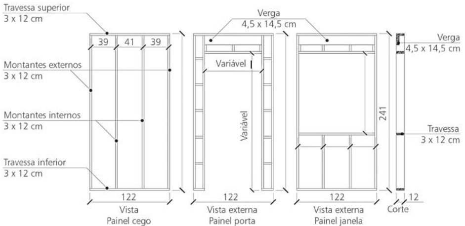
Figura 11: Detalhes dos painéis
