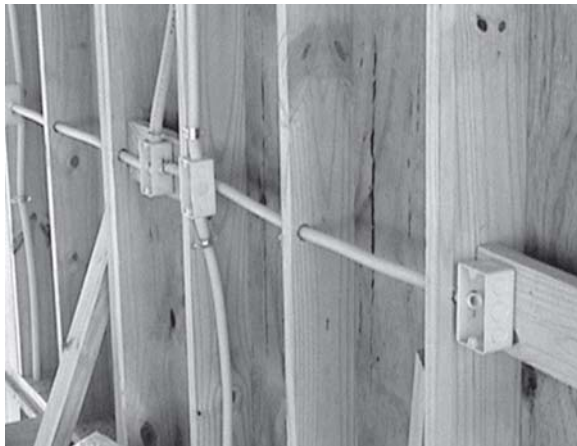
Figura 34: Eletrodutos flexíveis e caixas fixadas nos montantes
