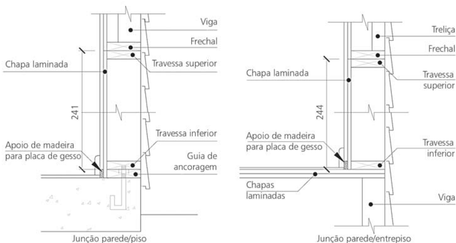
Figura 12: Detalhes de junção da parede com piso e com o entrepiso
