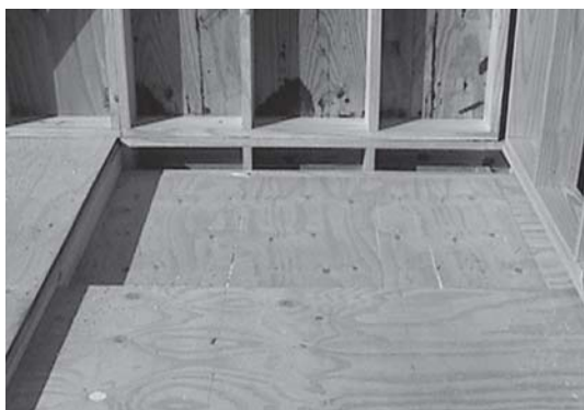
Figura 38: Piso em chapa de madeira com caimento do box
