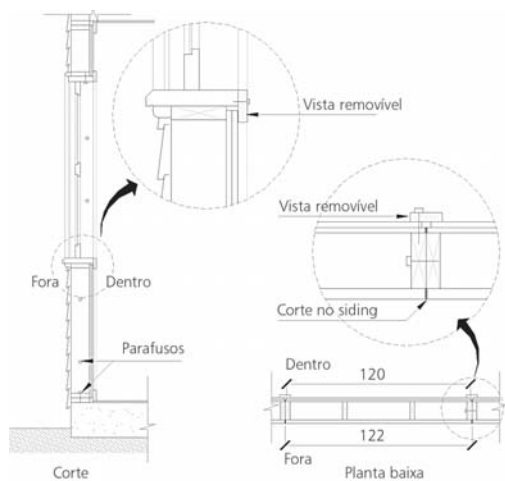
Figura 16: Solução para o painel removível
