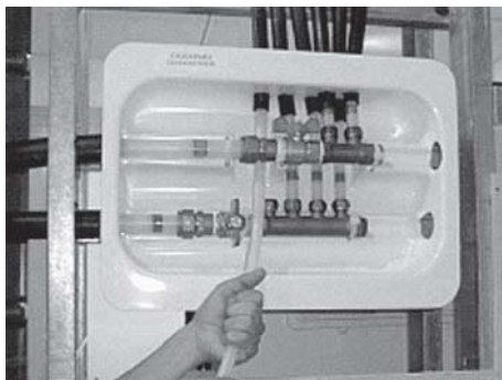
Figura 44: Instalação do quadro de distribuição ( www.pexdobrasil.com.br )
