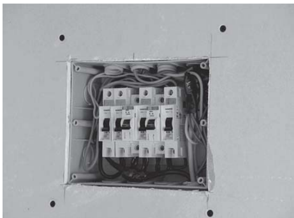
Figura 35: Caixa com disjuntores na ligação monofásica
